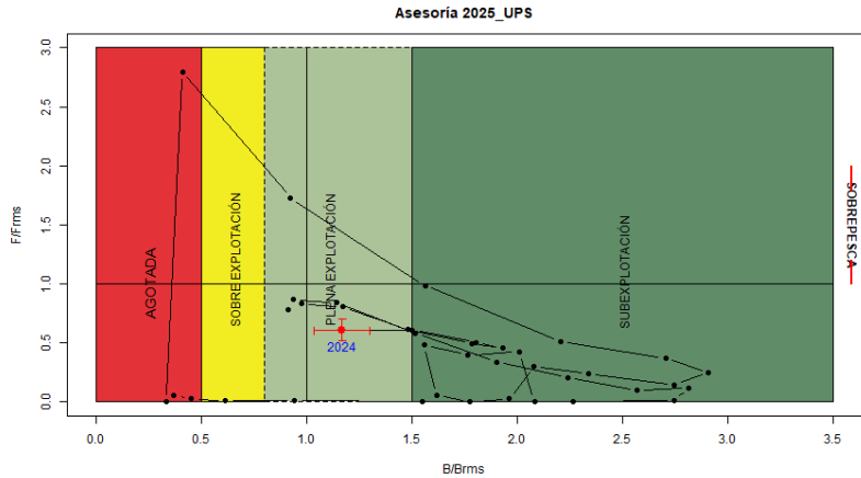
Diagrama de fases del recurso langostino colorado, en su Unidad de Pesquería Sur (UPS).
